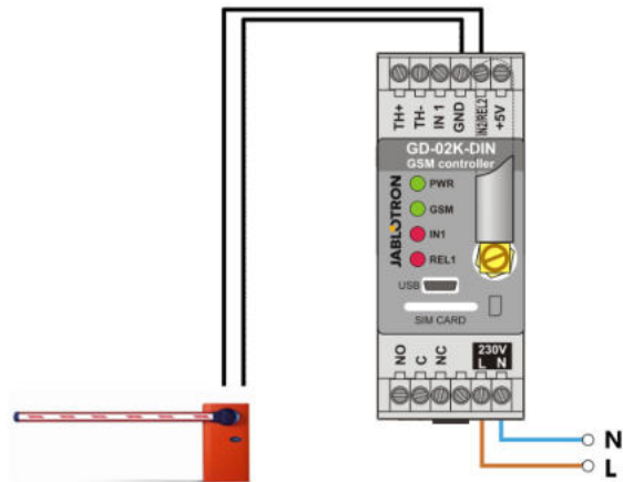
Abbildung 2: Tor-Controller GD-02K-DIN.
