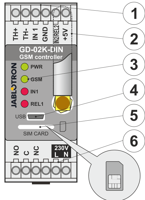
Abbildung 1: 1 – Niederspannungsklemmen; 2 – GSM-Antenne; 3 – LED-Anzeigen; 4 – MicroUSB-Anschluss zur Verbindung mit einem PC; 5 – SIM-Kartenfach; 6 – Stromausgangsrelaisklemmen und 230 V Stromklemmen.
