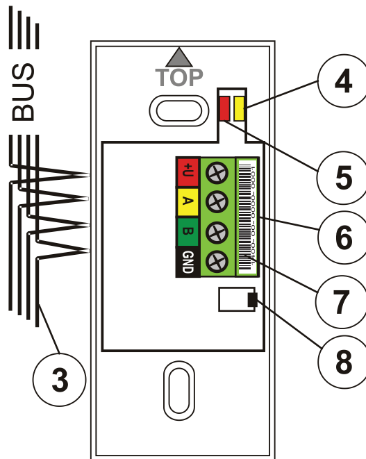
Abbildung: 3 – Kabel der Sammelleiste; 4 - gelbe Signallampe Störung; 5 – rote Signallampe Aktivierung; 6 – Klemmen der Sammelleiste; 7 - Seriennummer; 8 – Sabotageschalter
