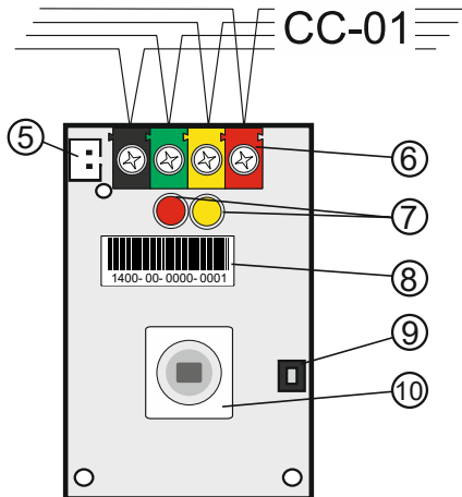
Abbildung 2: 5 – Anschluss für den externen Sabotage-Kontakt von JA-191PL, 6 – BUS-Klemmen, 7 – LED-Statusanzeigen, 8 – Seriennummer, 9 – Sabotagesensor der Abdeckung, 10 – PIR-Sensor
