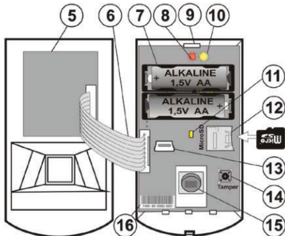
Abbildung: 5 – Kameramodul; 6 – Verbindungskabel; 7 – Batterien; 8 – rote LED-Anzeige; 9 – Lasche der Hauptplatte; 10 – gelbe LED; 11 – gelbe LED-Anzeige der Micro-SD-Karte; 12 – Micro-SD-Speicherkarte; 13 – miniUSB-Anschluss; 14 – Sabotagekontakt; 15 – PIR-Sensor; 16 – Seriennummer.
