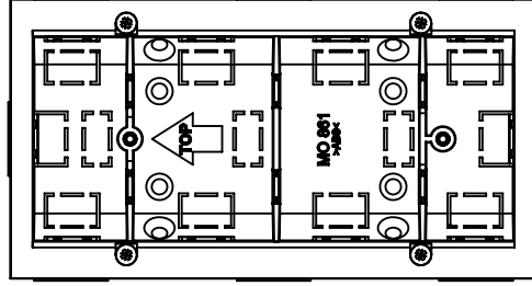
M Montážní otvor Mounting hole X=70/Y=136
