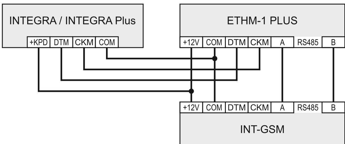
Abb. 7. Anschluss des Moduls INT-GSM an das Modul ETHM-1 Plus.
