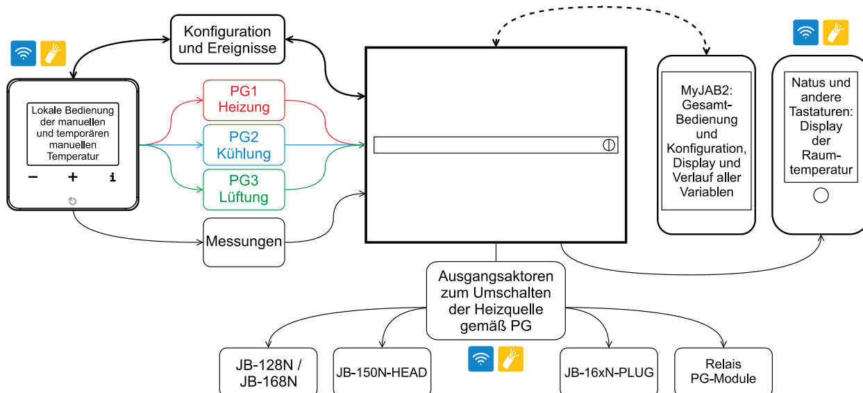
Abb. 4: Allgemeine Konfiguration der Bediengeräte für Heizung, Klimaanlage und Lüftung.
