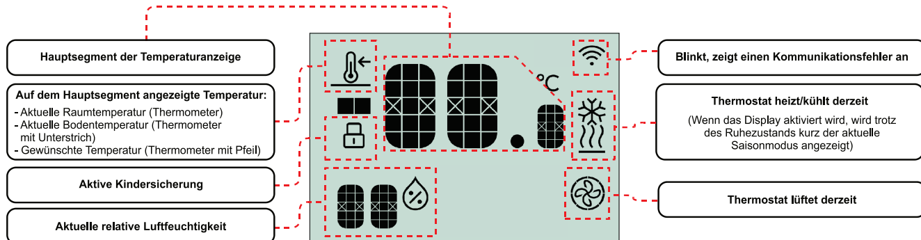
Abb. 5: Beschreibung der verschiedenen Display-Symbole auf dem Bildschirm
