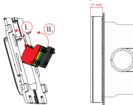
Abb. 3: Illustration einer teilweise versenkten Montage
