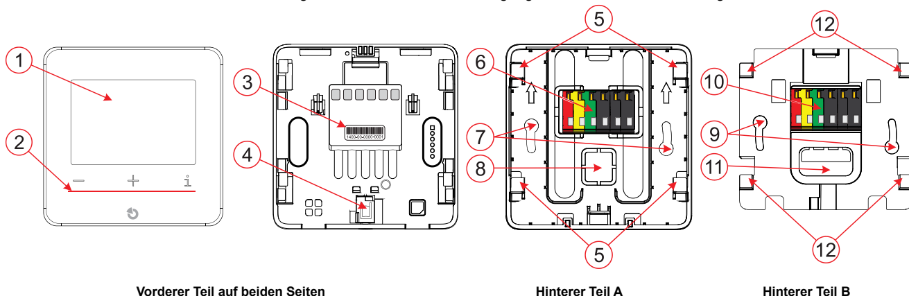
Abb. 1: Beschreibung der verschiedenen Teile des Produkts
