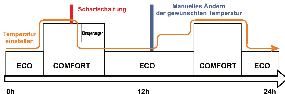
Abb. 6: Entwicklung der Temperaturen für einzelne Systemaktionen
