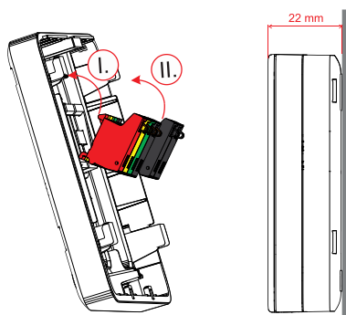
Abb. 2: Illustration der Aufputzmontage
